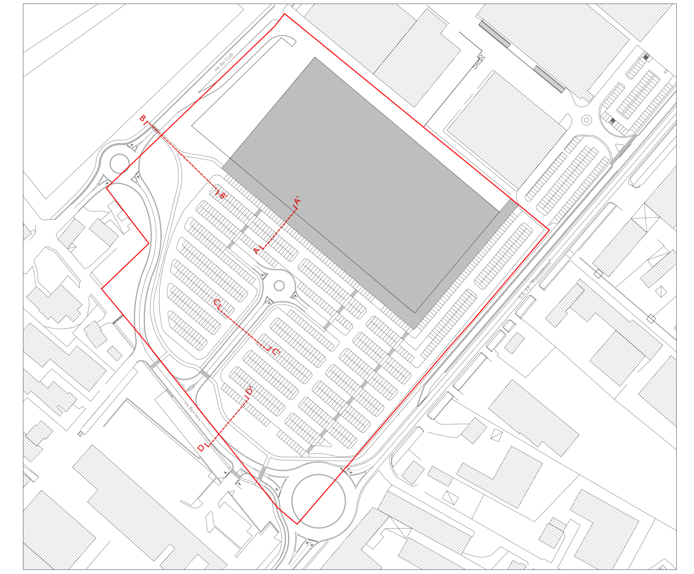
Planimetria con individuazione linee di sezione
