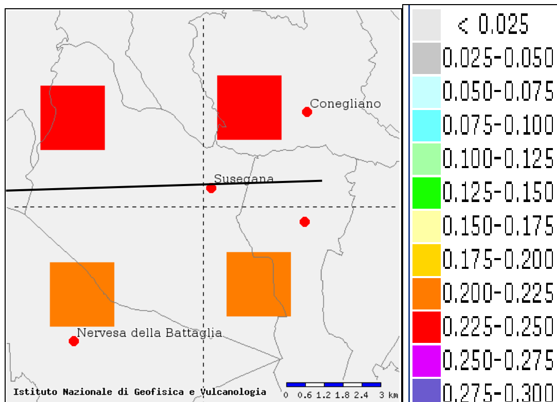
Fig. 9: Mappa di pericolosità sismica del territorio comunale di Sussejana
