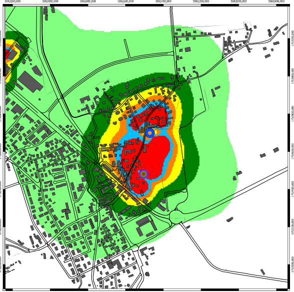
Campo elettromagnetico (V/m) calcolato alla quota di 17,7 m sul livello del terreno
