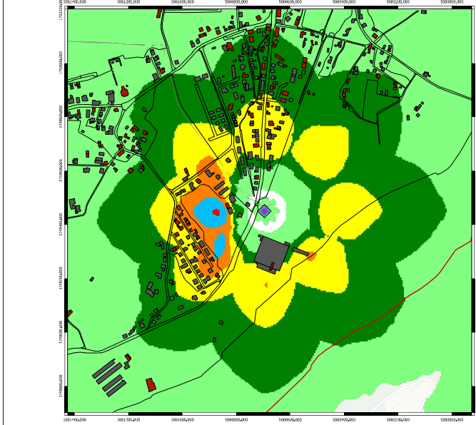
Campo elettromagnetico (V/m) calcolato alla quota di 7 m sul livello del terreno
