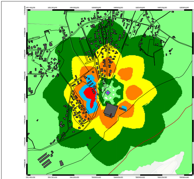
Campo elettromagnetico (V/m) calcolato alla quota di 11,7 m sul livello del terreno
