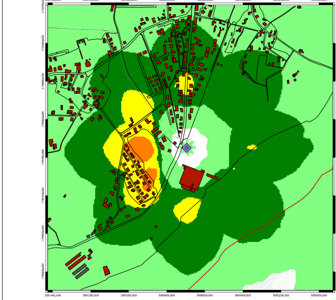
Campo elettromagnetico (V/m) calcolato alla quota di 2 m sul livello del terreno
