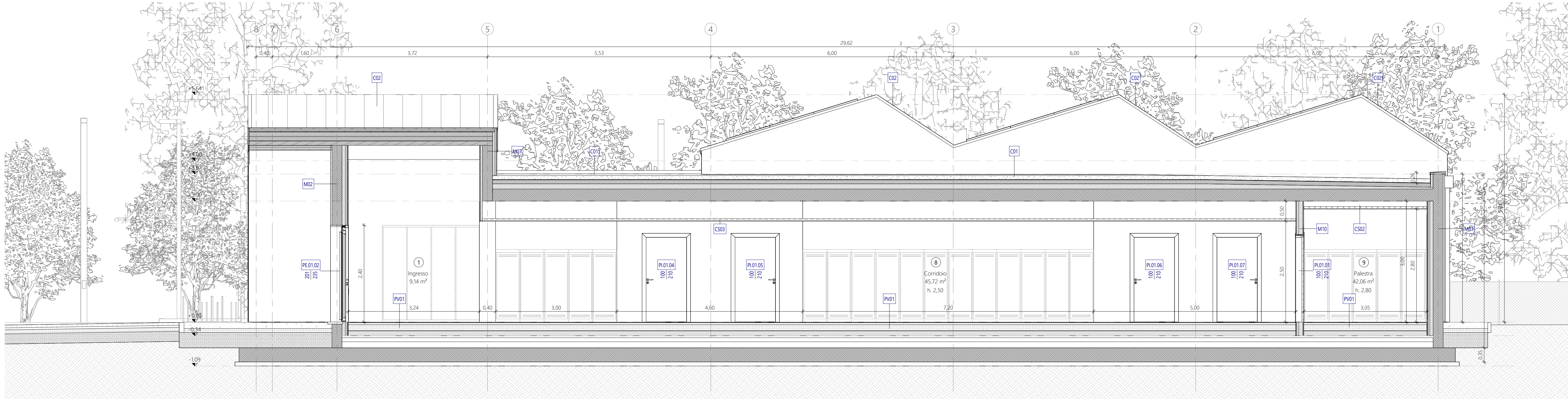
Sezione 2-2' - scala 1 : 50
