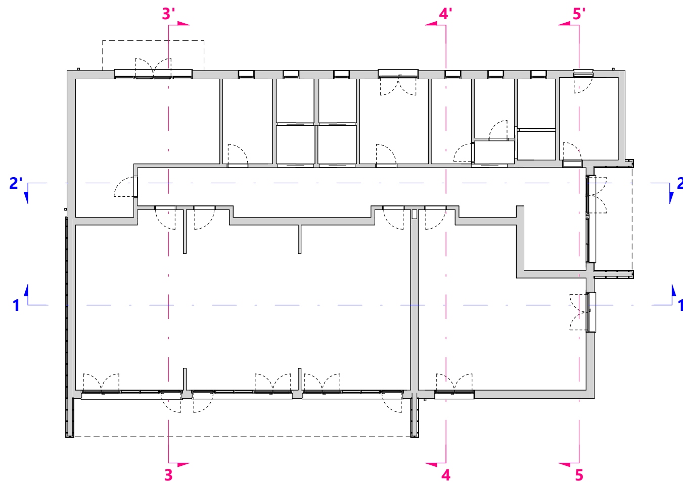
Keyplan - scala 1 : 200
