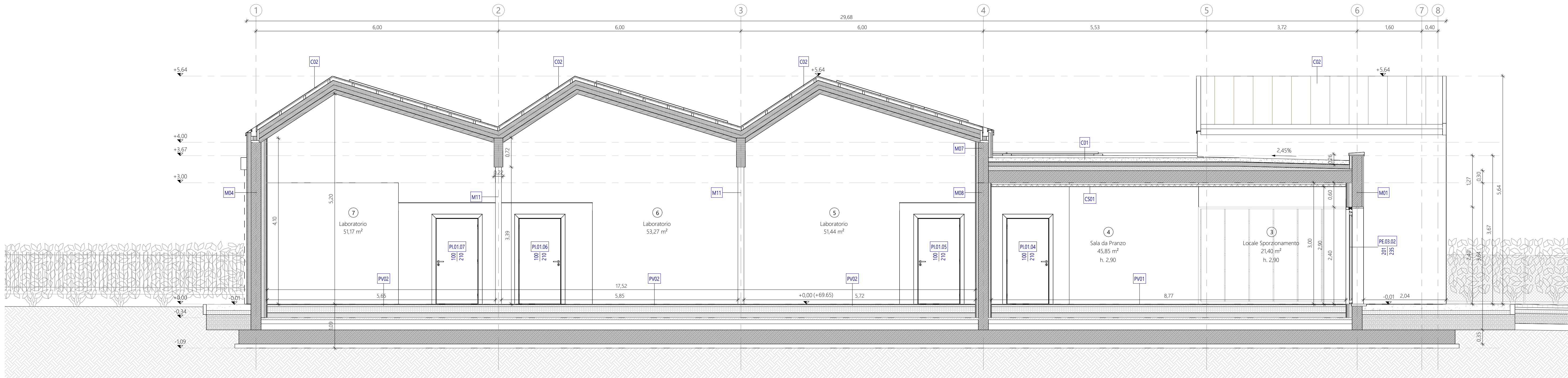
Sezione 1-1' - scala 1 : 50
