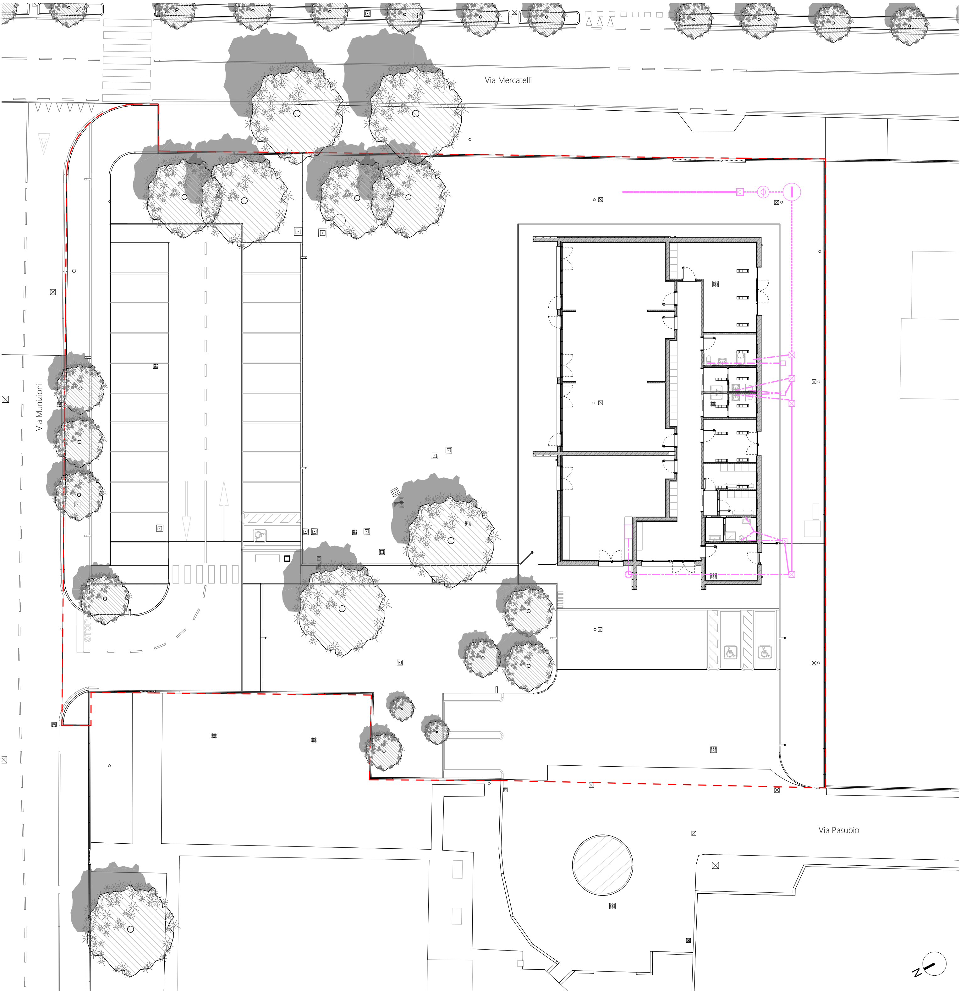
Attacco a terra - scala 1 : 200
